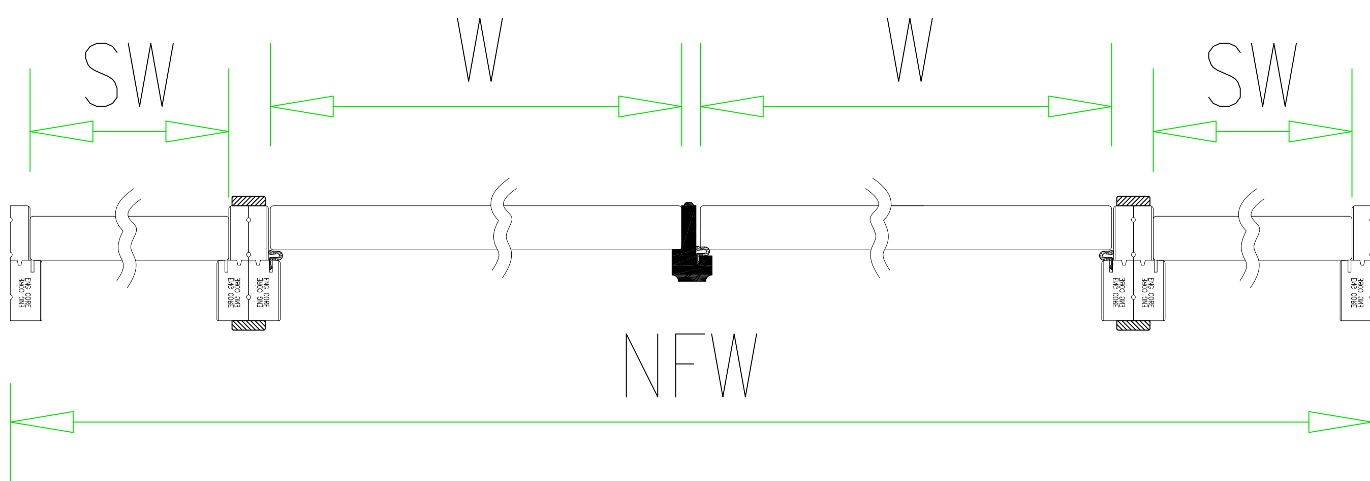
Double Door & Two Sidelites
